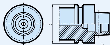
Form F – Teil 6 HSK-Größen 50 ... 80 Normentwurf
