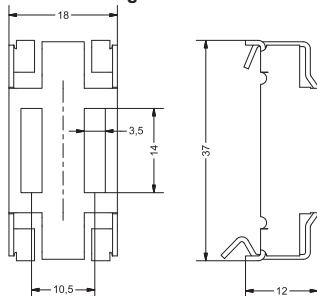
Maßzeichnung
