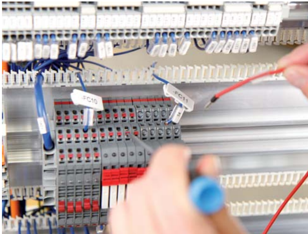
Schritt 1: Anschließen der Ader an der Komponente
