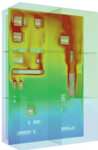
Freie Kühlung
