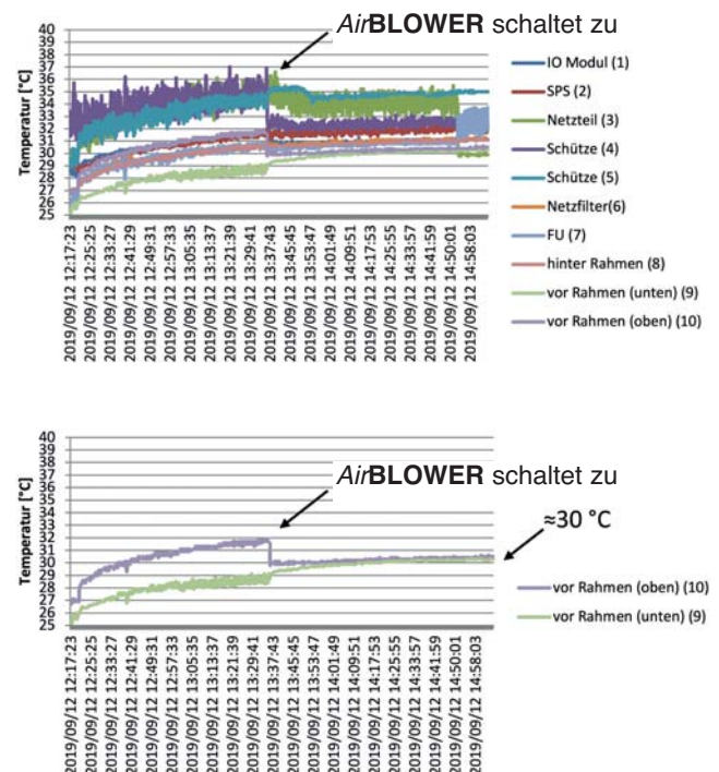
Abbildung 2: Temperaturen im Schaltschrank bei geregelterm AirBLOWER -Betrieb
