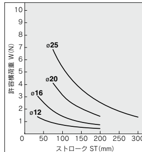
〈図5〉ロングストローク / オートスイッチなし・付
