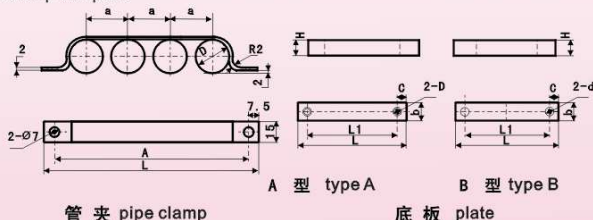
管夹 pipe clamp
