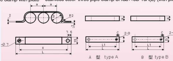
管 夹 pipe clamp
