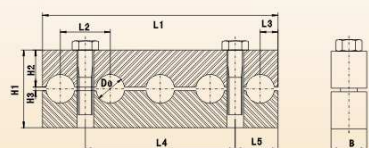
管夹 pipe clamp 底板 plate
