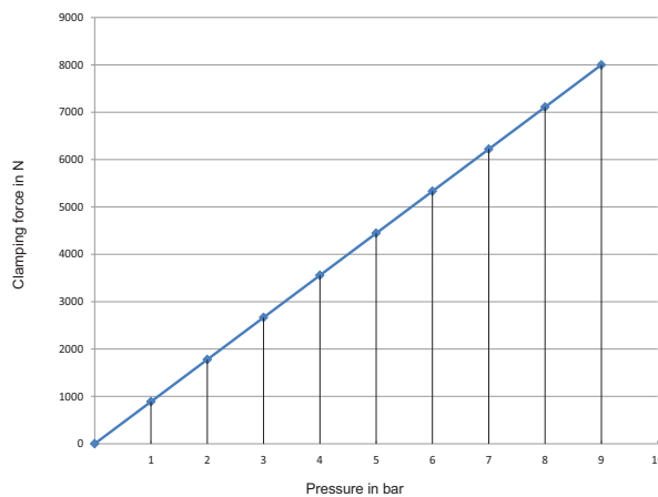
Diagramme clamping force BSPD-64
