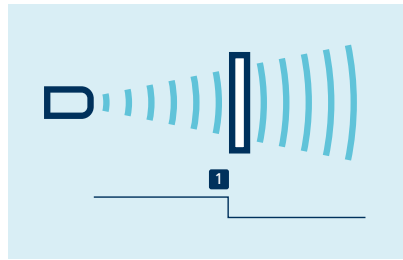
Teach-in eines Schaltpunktes
