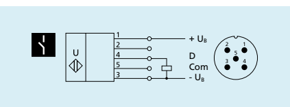
1 pnp-Schaltausgang
