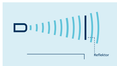
Teach-in einer Zweiweg-Reflexionsschranke
