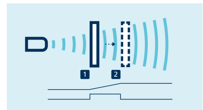
Teach-in einer Analogkennlinie bzw. eines Fensters mit zwei Schalterpunkten
