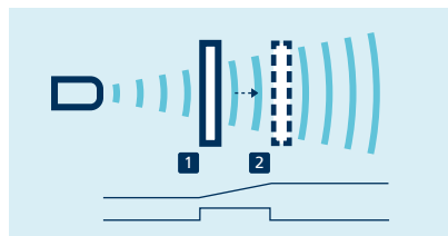
Teach-in einer Analogkennlinie bzw. eines Fensters mit zwei Schalterpunkten
