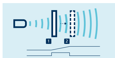
Teach-in einer Analogkennlinie bzw. eines Fensters mit zwei Schaltpunkten
