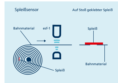
esf-1 als Spleißsensor
