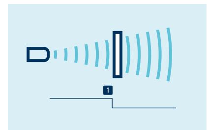
Teach-in eines Schaltpunktes
