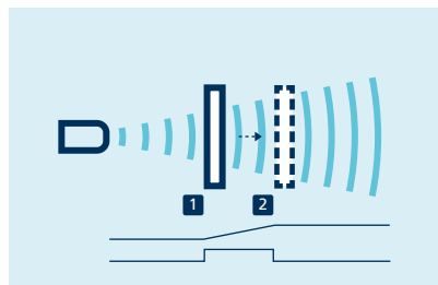
Teach-in einer Analogkennlinie bzw. eines Fensters mit 2 Schaltpunkten
