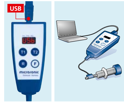
USB-Schnittstelle für den Anschluss an einen PC
