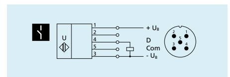
1 pnp-Schaltausgang
