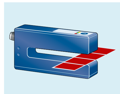
Die Etiketten werden durch die Gabel geführt. Der esf-1 reagiert auf den Signalunterschied zwischen Trägermaterial und Etikett.
