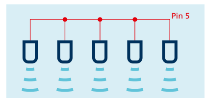
Synchronisation über Pin 5
