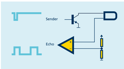
Kundenseitige Ansteuerung eines wms Sensor
