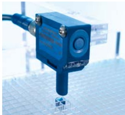
Mit der SoundPipe misst der zws-15 Sensor Füllstände in kleinsten Öffnungen.
