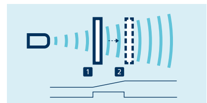
Teach-in einer Analogkennlinie bzw. eines Fensters mit zwei Schalterpunkten
