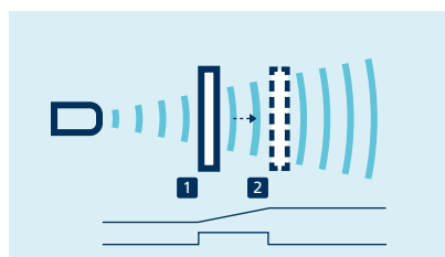
Teach-in einer Analogkennlinie bzw. eines Fensters mit zwei Schalterpunkten
