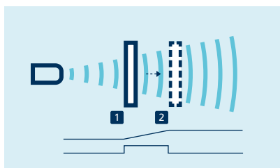
Teach-in einer Analogkennlinie bzw. eines Fensters mit zwei Schaltpunkten
