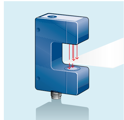
Mit einer Gabelbreite von nur 30 mm und einer Tiefe von 33 mm ist er sehr kompakt gebaut. Der Arbeitsbereich von 8 mm und die hohe Genauigkeit von 0,1 mm erlauben einen vielfältigen Einsatz.
