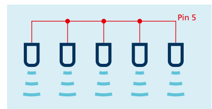
Synchronisation über Pin 5
