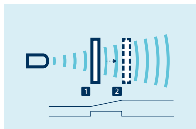
Teach-in einer Analogkennlinie bzw. eines Fensters mit zwei Schaltpunkten
