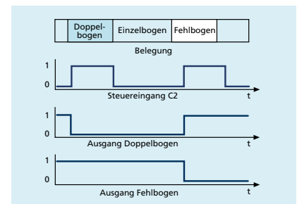
Trigger-Mode – pegelgesteuert
