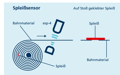
esp-4 als Spleißsensor
