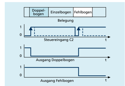
Trigger-Mode – flankengesteuert
