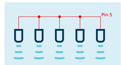
Synchronisation über Pin 5
