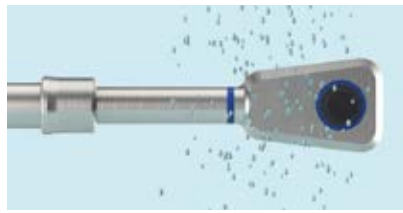
Robuster Edstahlsensor im Hygienic Design, alle waagerechten Flächen sind mindestens 3^\circ geneigt
