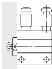
取付状態3
